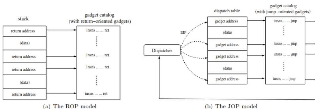
Figura 2.5: Diferencias entre las técnicas ROP y JOP.
